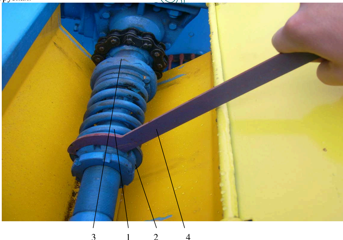
Рис. 3 – муфта предохранительная.
