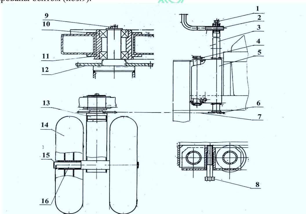
Рисунок 5.9 Рулевой механизм:
