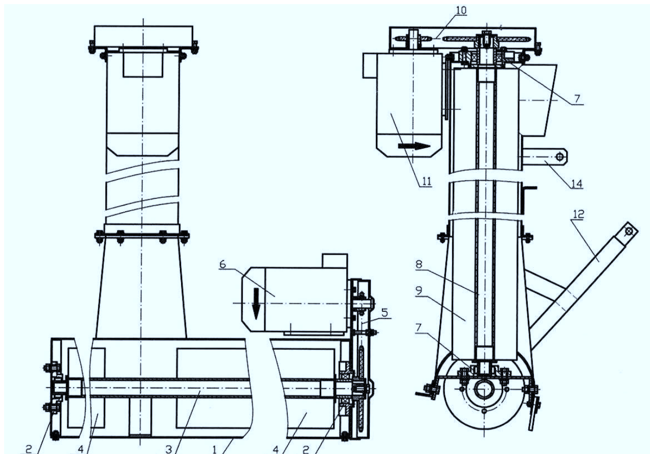
Рисунок 5.2 Загрузочный шнек:
