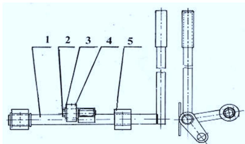
Рисунок 5.8 Механизм подъема загрузочного шнека:
