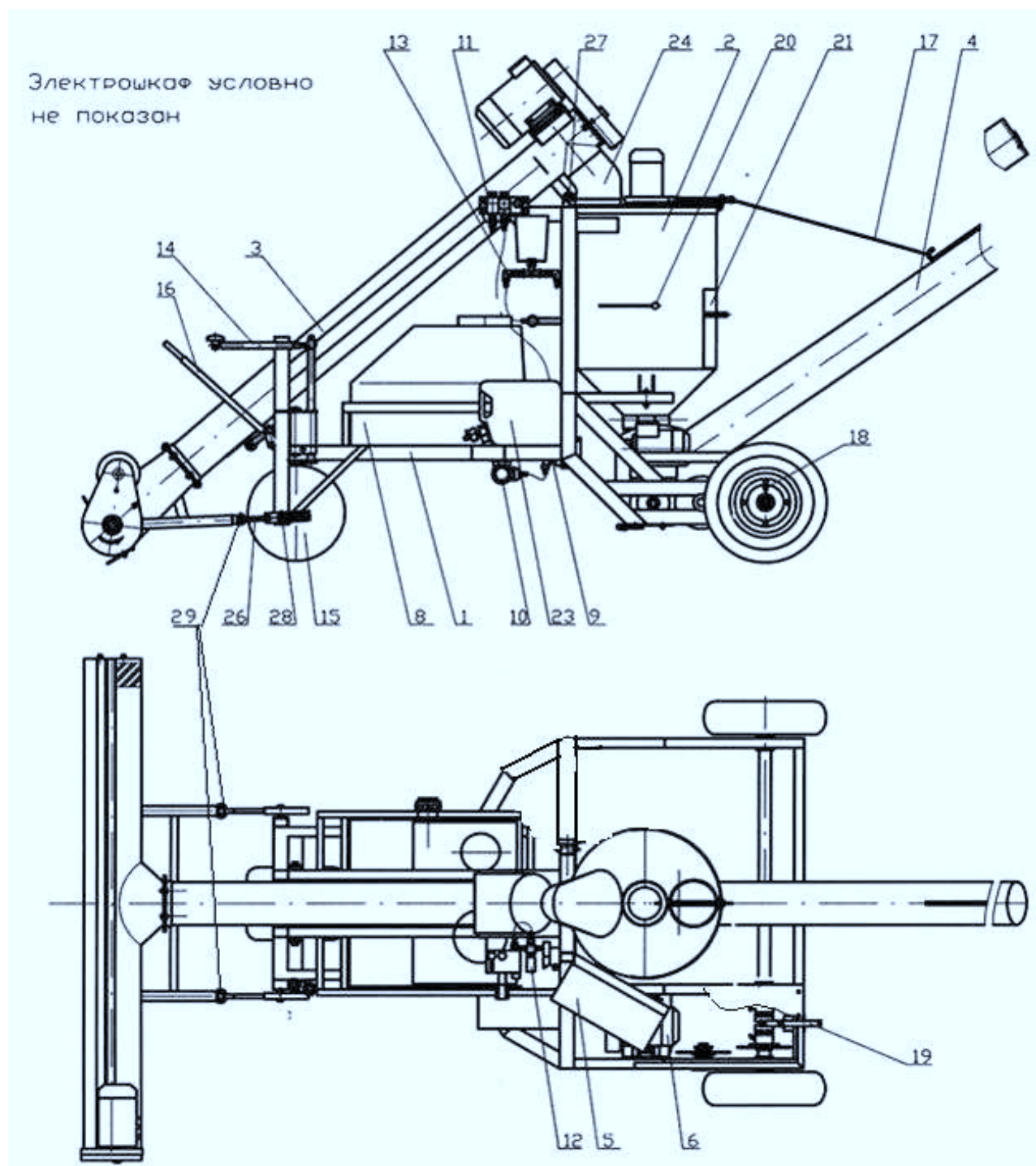
Рисунок 4.1 Протравливатель семян камерный ПСК-15. Основные сборочные единицы и органы управления:
