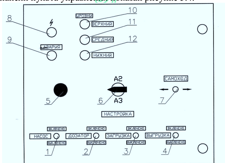
Рисунок 5.4 Панель пульта управления:
