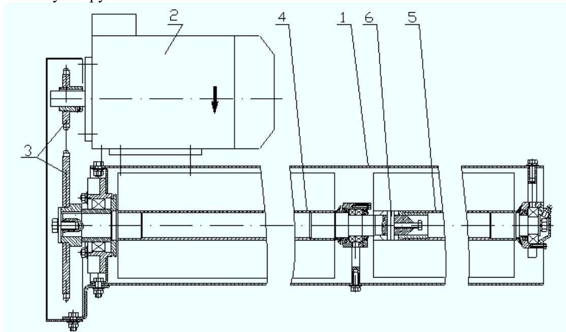
Рисунок 5.3 Конструкция выгрузного шнека:
