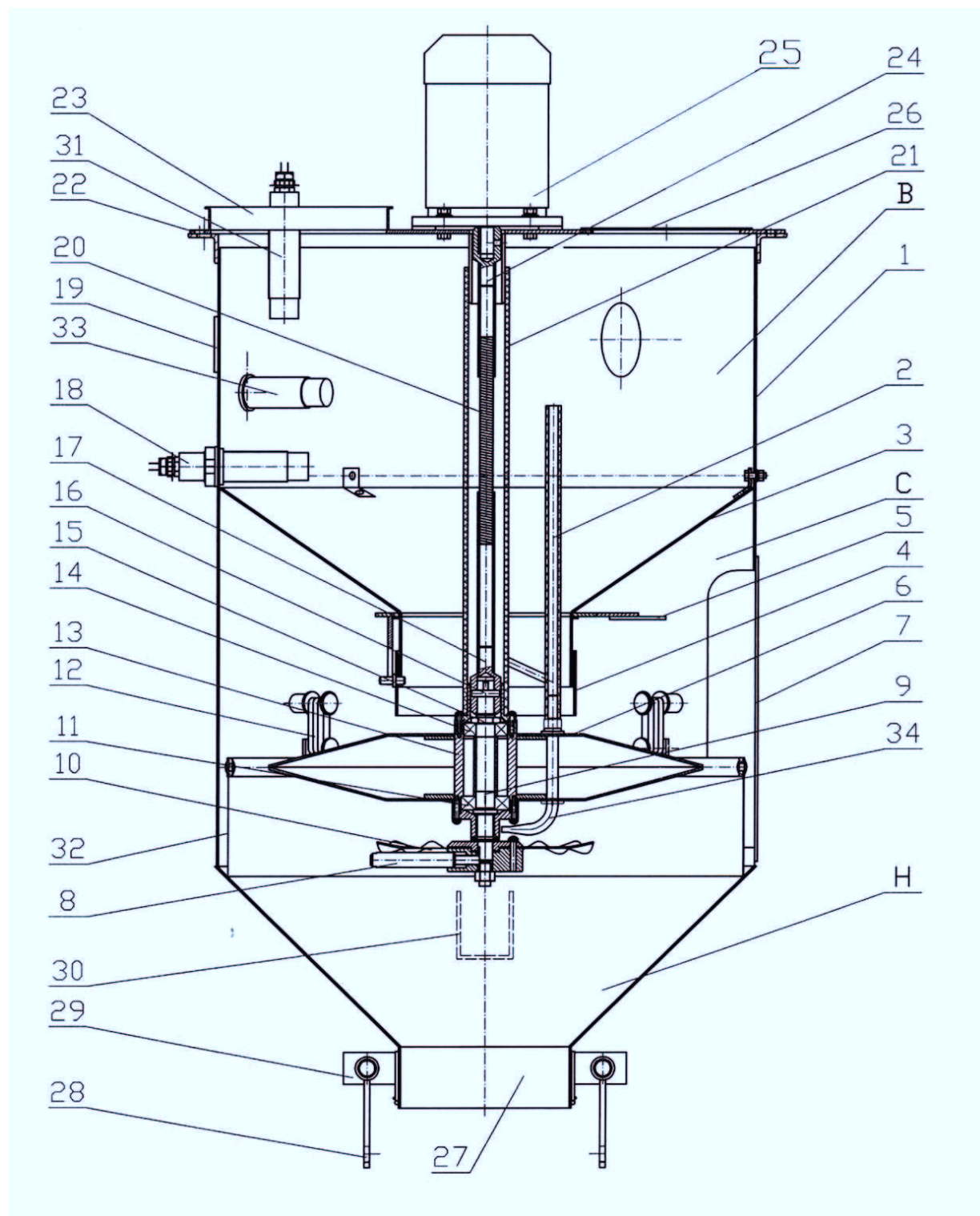
Рисунок 5.1 Модуль дозированного смешивания (МДС):
