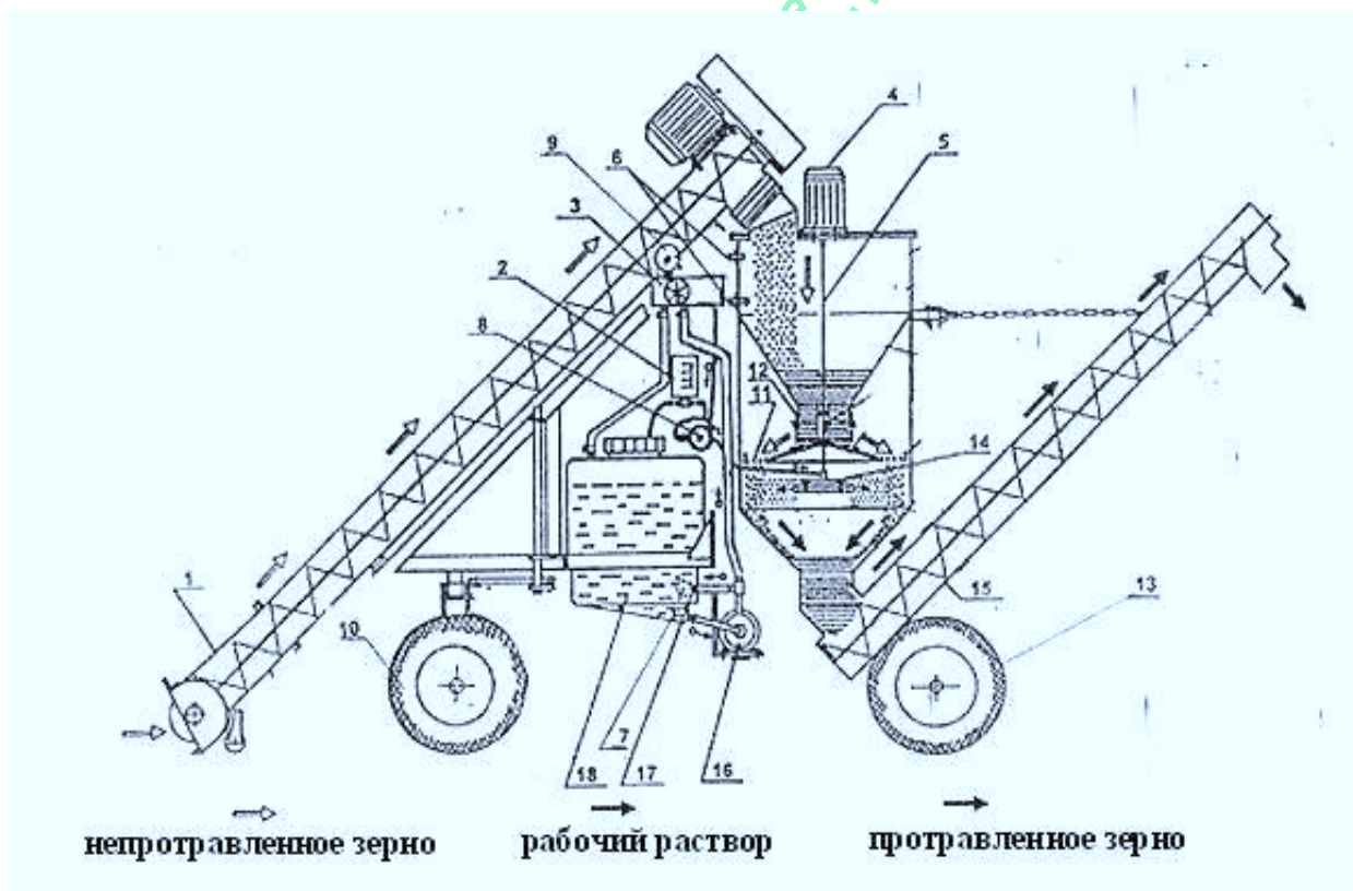
Рисунок 4.2 Технологическая схема протравителя.
